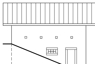
Prospecto laterale
