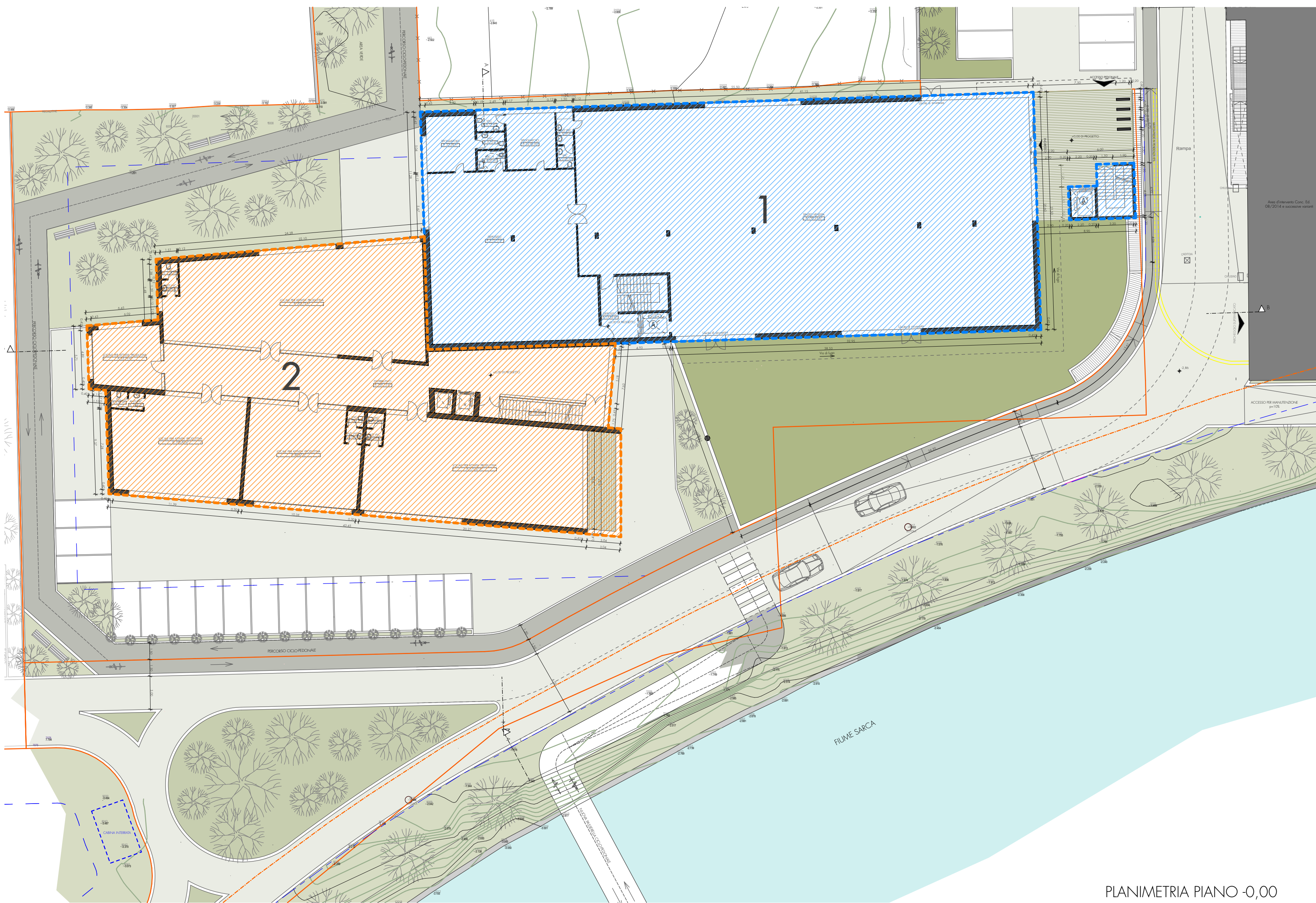
PLANIMETRIA PIANO -0,00
